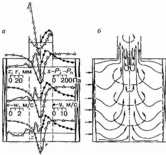
Рис. 2. Профили скорости и давления (а) и схема течения (б) в боковой камере с боковым вдувом.
