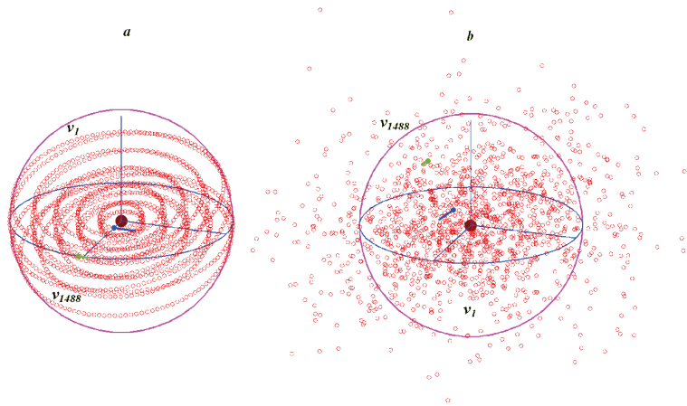
Рис. 1. Многослойная сферическая модель шарового звездного скопления: показаны пять слоев, включающих 1488 периферийных тел; а – в момент формирования многослойной структуры; б – после 196-го обращения тела первого слоя; отрезками у тел 1 и 1488 показаны их векторами скорости: v_1 и v_{1488} .
